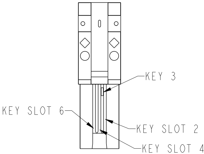
KEY 3 & KEY SLOT 2,4 & 6 ○◇ UNIVERSAL PORT END P2 & END P3 MINI SAS
