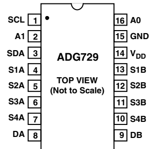
ADG729
