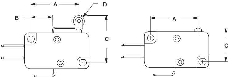
FIG. 1 Lever Roller FIG. 2 Pin Roller
