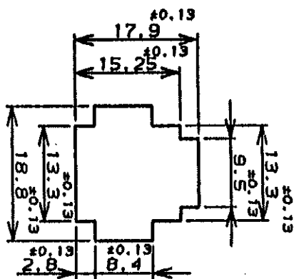
コネクタ取付寸法 FIG. 1 (RECOMMENDED PANEL OPENING DIMENSION)
