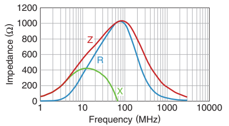
KMZ1608RHR102ATD25
