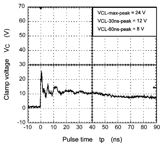
Fig. 9.1 +8 kV
