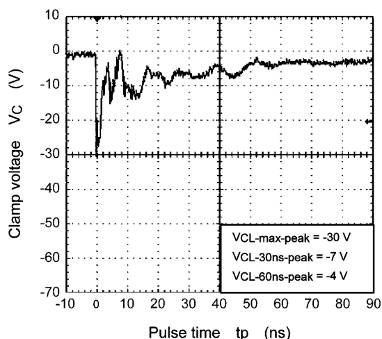
Fig. 9.4 -15 kV
