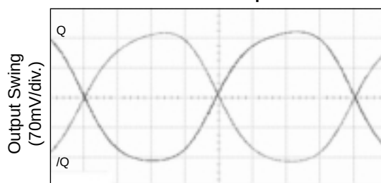
2.5GHz Output
