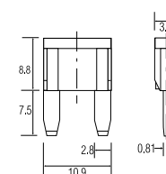
MINI dimensions in mm
