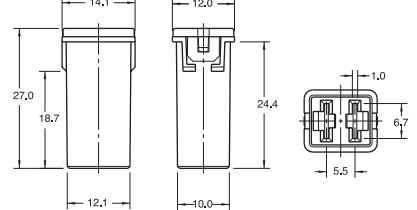
Dimensions JCASE®
