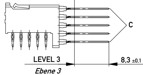
DATUM PLANE DEPTH Bezugsebene Tiefe
