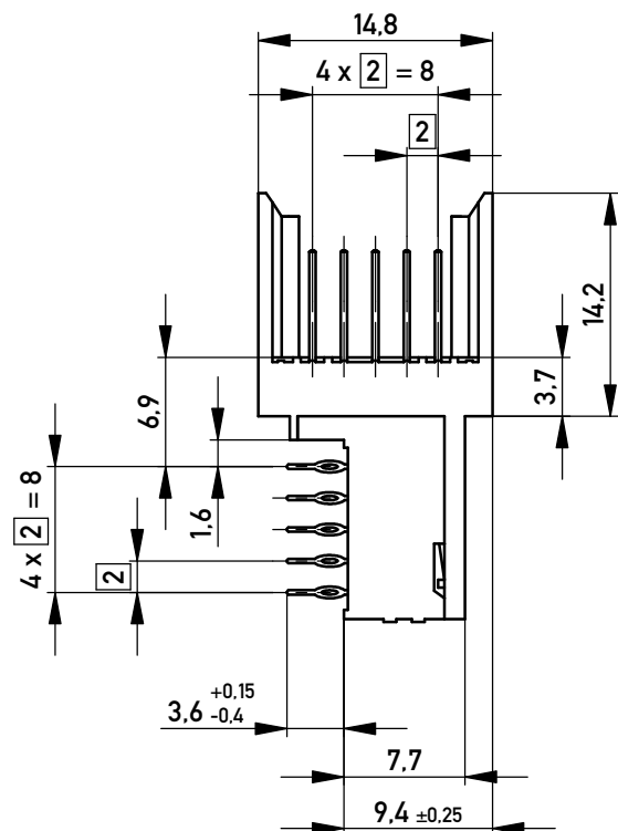
CONTACT LENGTH EXAMPLES Kontaktlänge Beispiele
