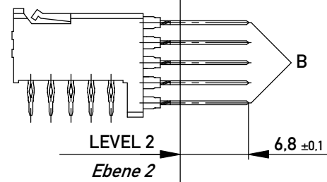
DATUM PLANE DEPTH Bezugsebene Tiefe
