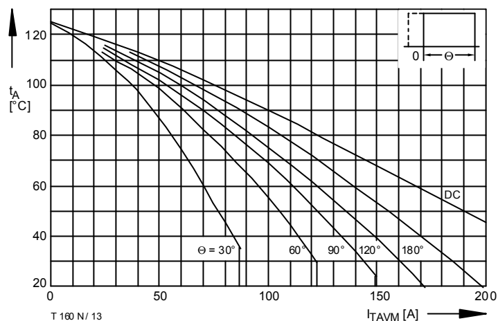
Bild / Fig. 13 Höchstzulässige Kühlmitteltemperatur / Max. allowable cooling medium temperature t_A = f(I_{TAVM}) Verstärkte Luftkühlung / Forced air-cooling, V_L = 50 \text{ l/s} Kühlkörper / Heatsink: K0.55-M12-A, V_L = 50 \text{ l/s} Parameter: Stromflußwinkel / Current conduction angle \theta
