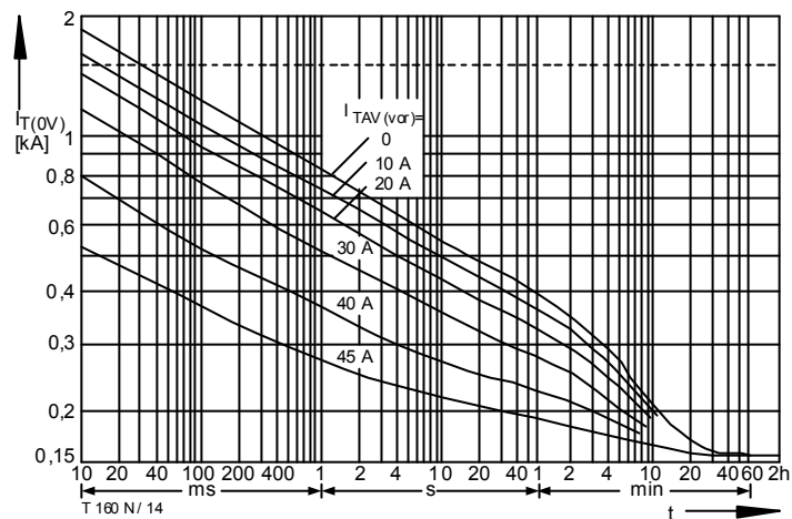
Bild / Fig. 15 Überstrom / Overload on-state current I_{T(OV)} = f(t) Verstärkte Luftkühlung / Forced air-cooling, t_A = 35^\circ\text{C} Kühlkörper / Heatsink: K0.11-M12-A, V_L = 30 \text{ l/s} Parameter: Vorlaststrom / Pre-load current I_{TAV(vor)}
