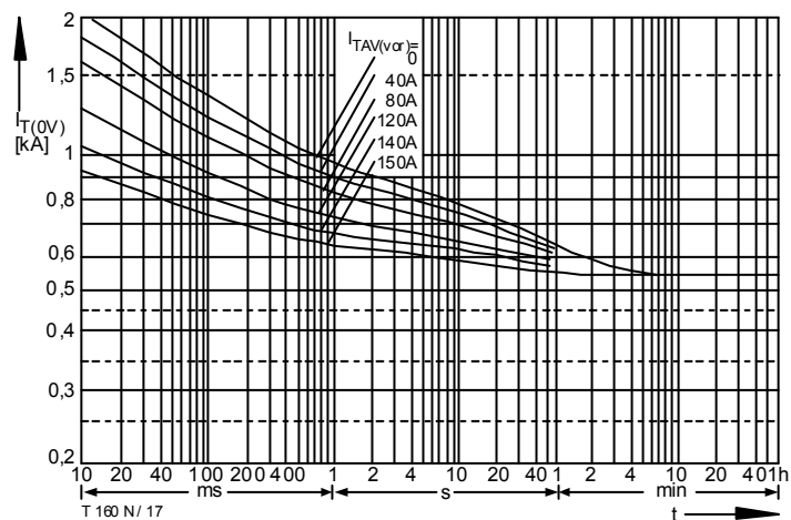
Bild / Fig. 17 Überstrom / Overload on-state current I_{T(OV)} = f(t) Verstärkte Luftkühlung / Forced air-cooling, t_A = 35^\circ\text{C} Kühlkörper / Heatsink: K0.55-M12-A, V_L = 50 \text{ l/s} Parameter: Vorlaststrom / Pre-load current I_{TAV(vor)}
