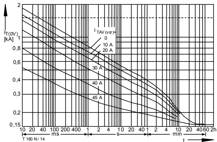
Bild / Fig. 15 Überstrom / Overload on-state current I_{T(OV)} = f(t) Verstärkte Luftkühlung / Forced air-cooling, t_A = 35 °C Kühlkörper / Heatsink: K0.11-M12-A, V_L = 30 l/s Parameter: Vorlaststrom / Pre-load current I_{TAV(vor)}
