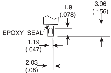
SOLDER LUG
