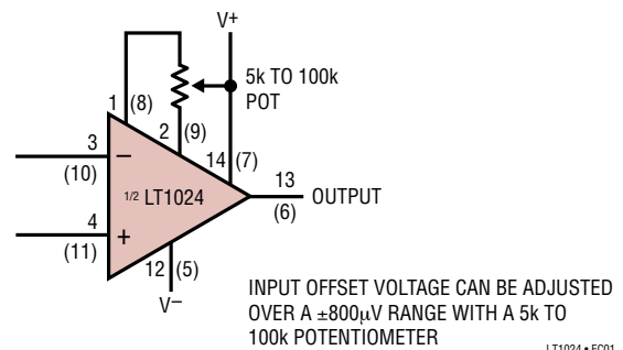
Optional Offset Nulling Circuit
