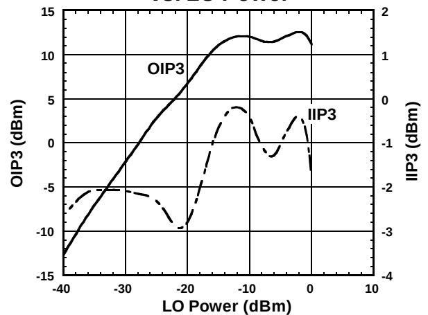
Output IP3 , Input IP3 vs. LO Power
