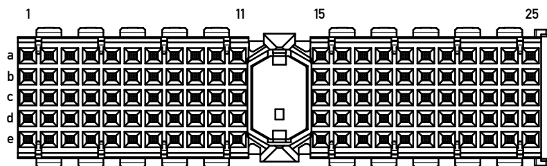
Bestückungsplan / contact layout
