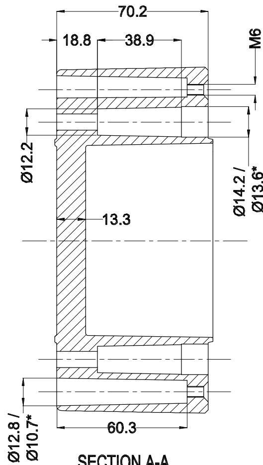
SECTION A-A
