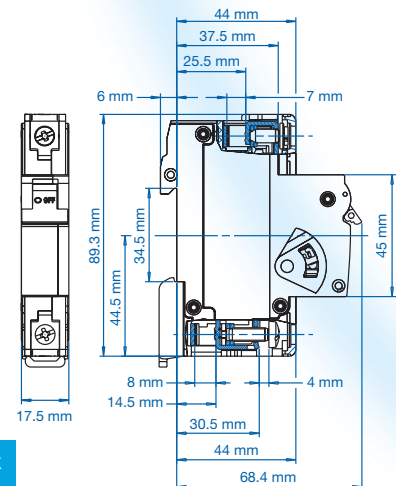
Dimensions N63UM, FxaxxUM.
