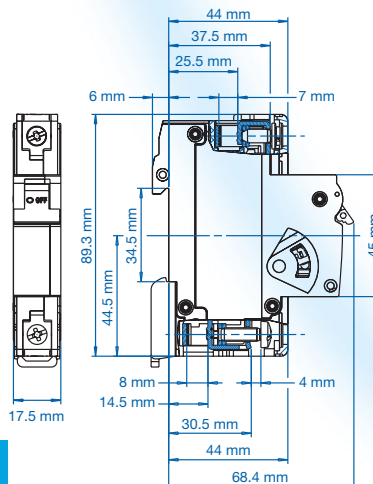
Dimensions N63UM, FxXXUM.
