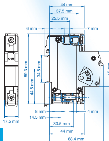
Dimensions N63UM, FxXXUM.
