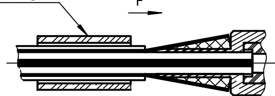
FERRULE
