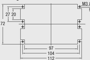
Montageausschnitt/Panel cut-out
