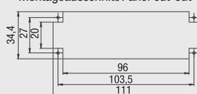
Montageausschnitt/Panel cut-out
