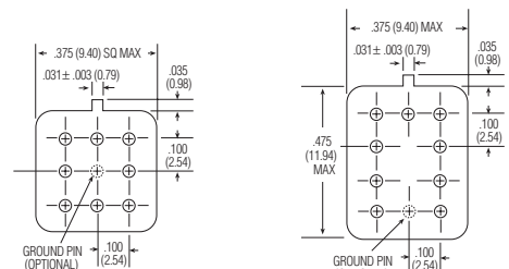
MGS/MGSD/MGSDD HEADER
