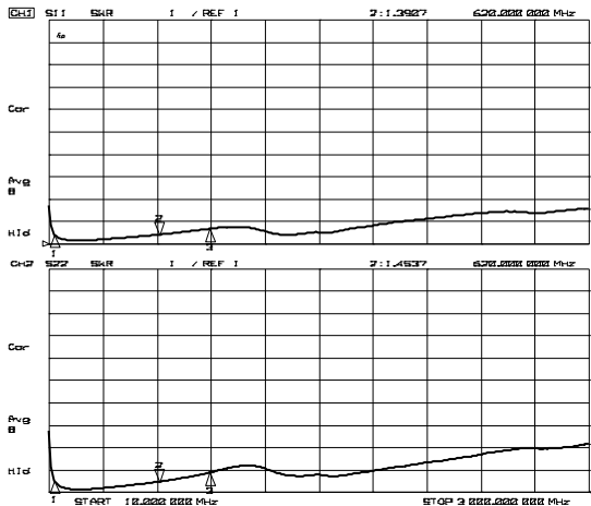
VSWRi, VSWRo
