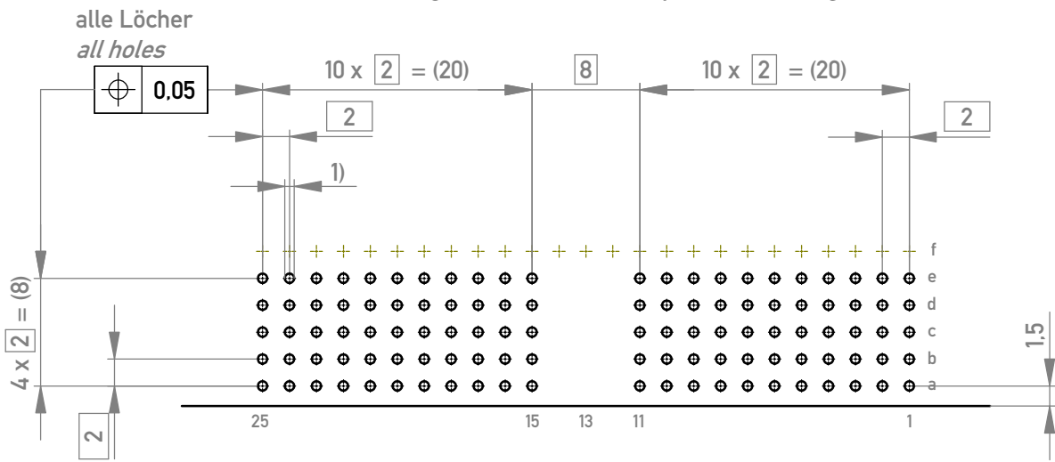
Lochbild für Leiterplatte (Bestückungsseite)
