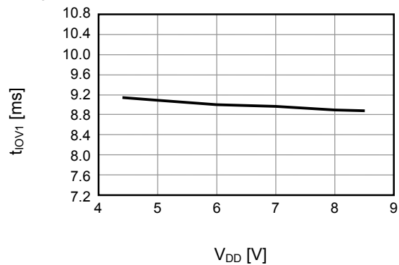
11. t_{IOV1} - V_{DD}
