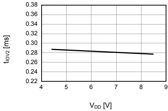
13. t_{IOV2} - V_{DD}
