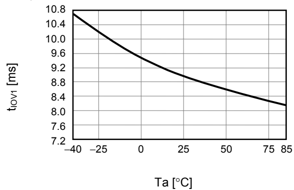
12. t_{IOV1} - T_a
