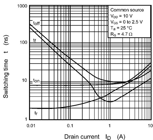
Fig. 7.11 t - I_D
