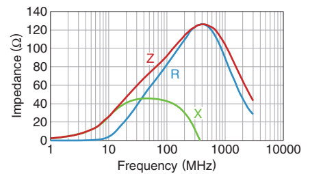
MMZ2012S301ATD25
