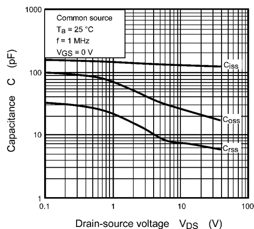
Fig. 7.10 C - V_{DS}
