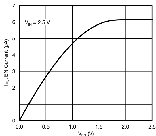
EN Input Leakage vs. V_{EN}
