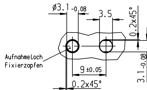
Empfohlenes Lochbild
