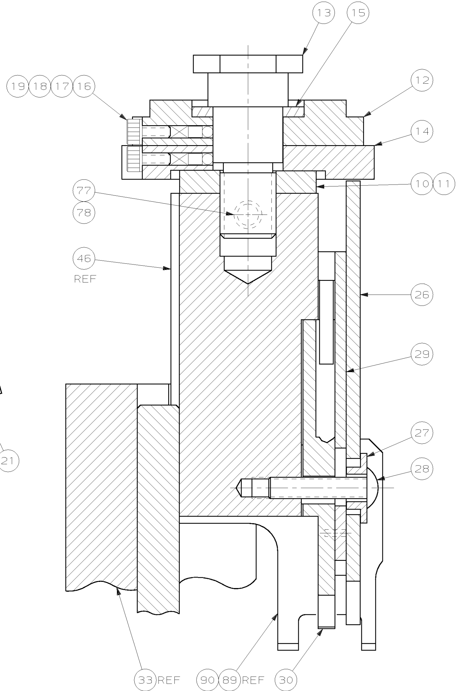
SECTION D-D SCALE 2:1
