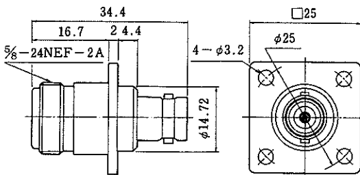
SJ-BNCJ-PA(40)
