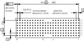
Lochbild für Leiterplatte (Bestückungssite) Board hole pattern (Component mounting side)
