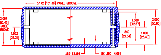
SECTION A-A LH57-200
