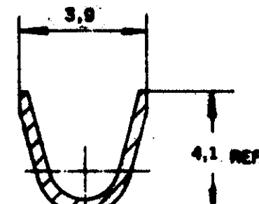
SEÇÃO B-B
